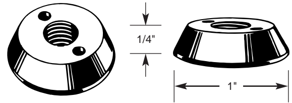
Spanner Nuts
